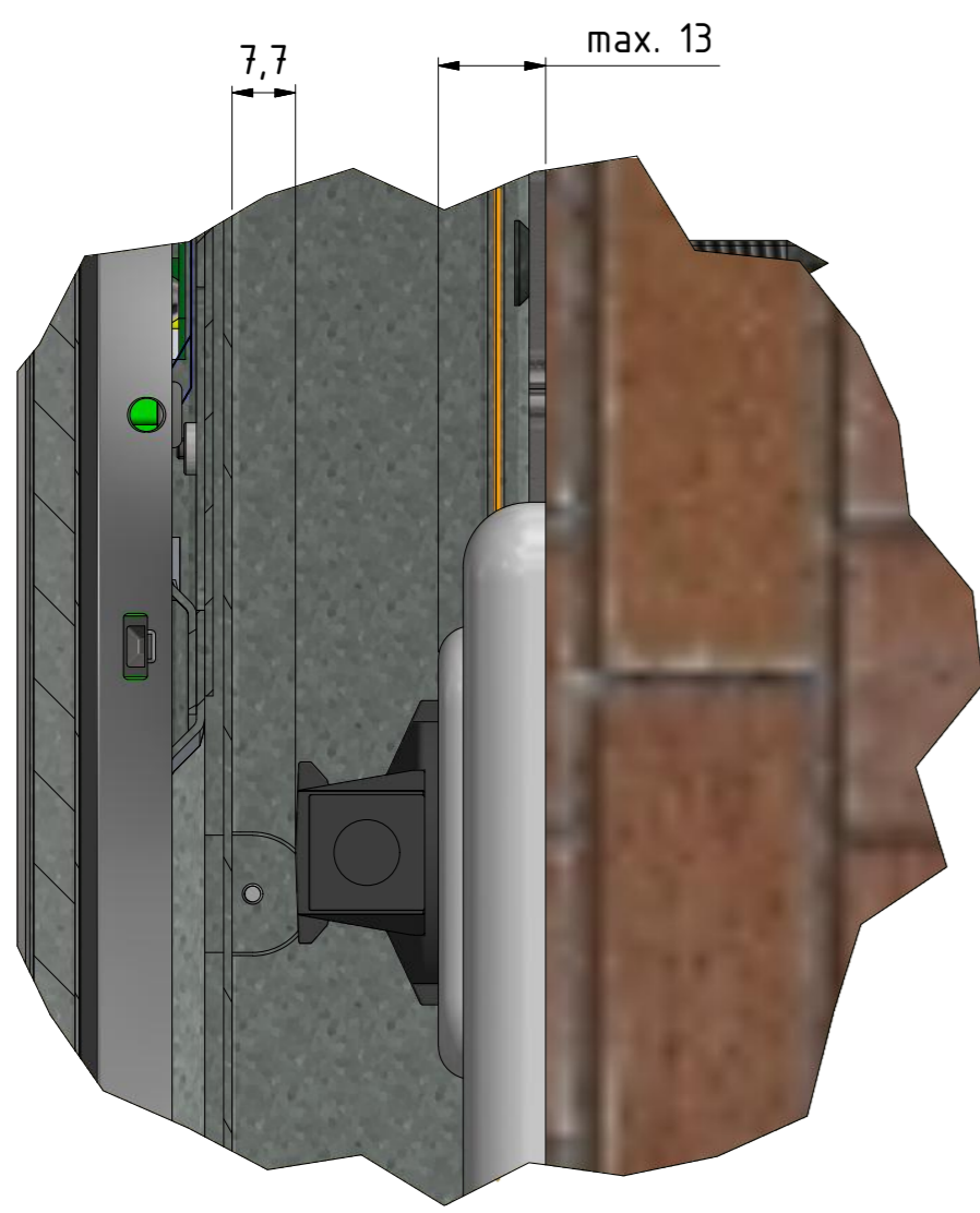
F ( 1 : 1 )
